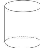
Cilindro
