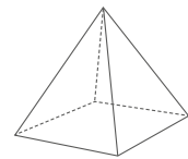
Pirámide cuadrada
