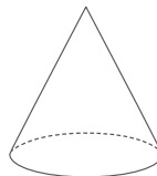
Cono
